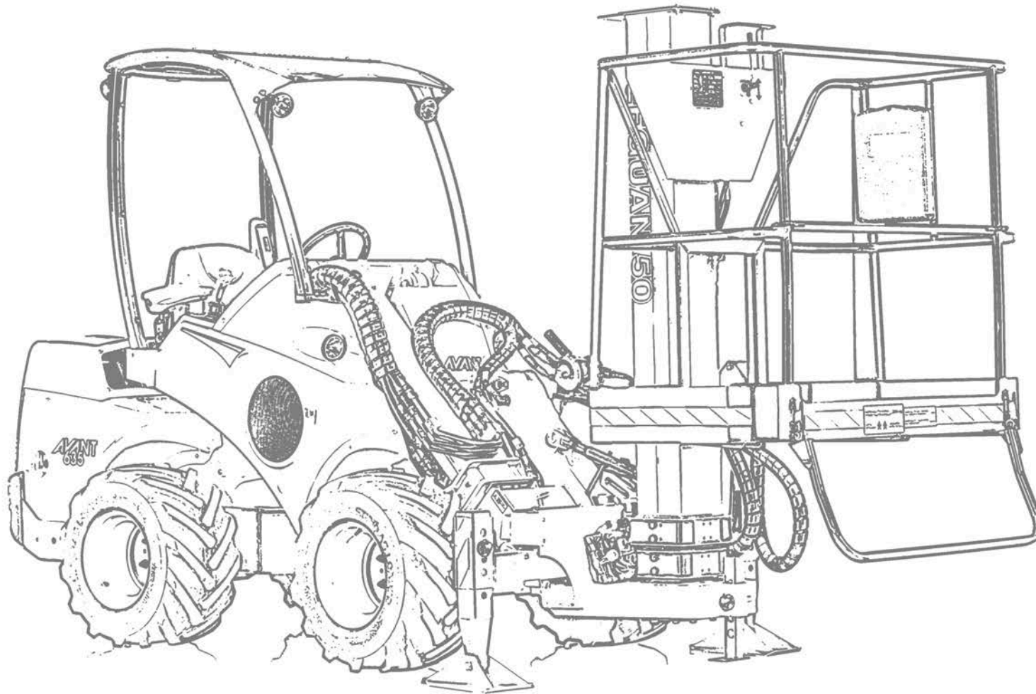
podnośnik koszowy Leguan 50
